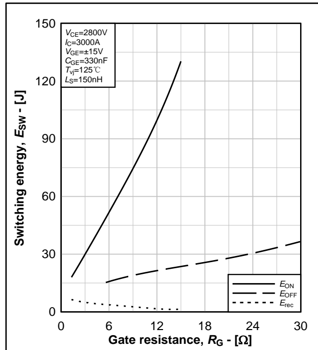
图 6. IGBT 及 FRD 开关能耗典型曲线,
