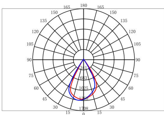
配光曲线
