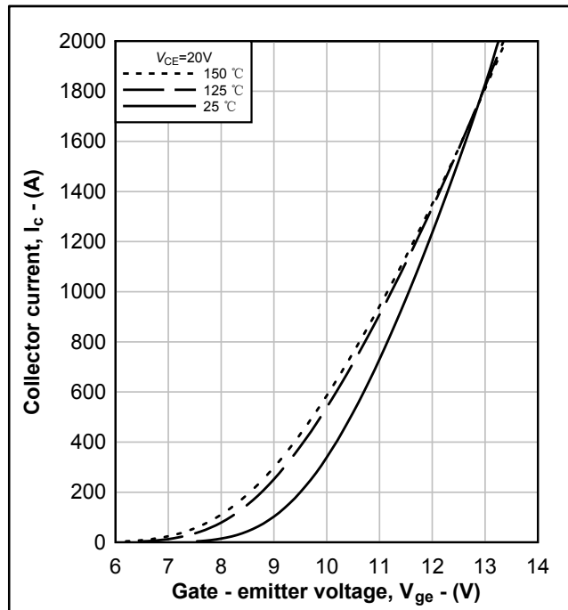
图 6. IGBT 传输特性典型曲线, I_c = f(V_{GE})
