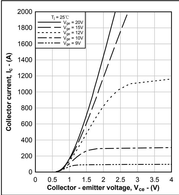
图 3. IGBT 输出特性典型曲线, I_c = f(V_{CE})
