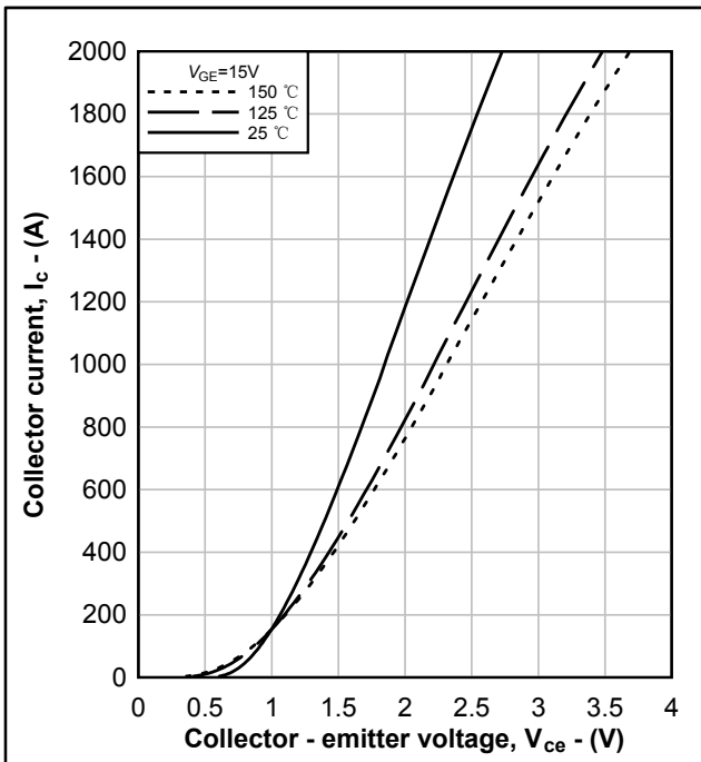
图 5. IGBT 输出特性典型曲线, I_c = f(V_{CE})
