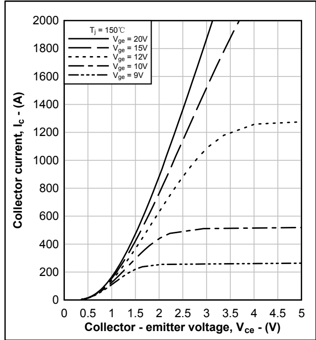
图 4. IGBT 输出特性典型曲线, I_c = f(V_{CE})
