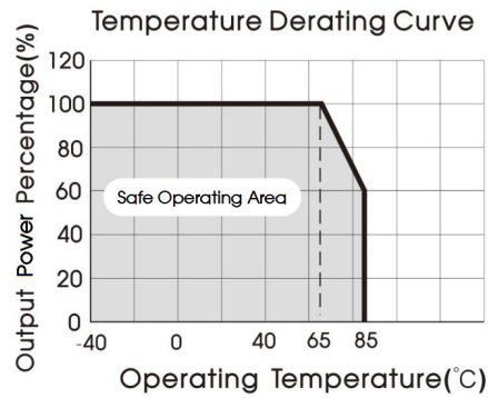
Fig. 1 (Vin=48V)
