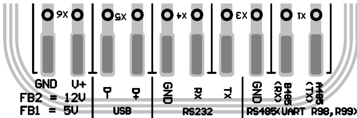
Рис.1 Подключение считывателя UEM Mifare/ICode/NFC RS wall reader
