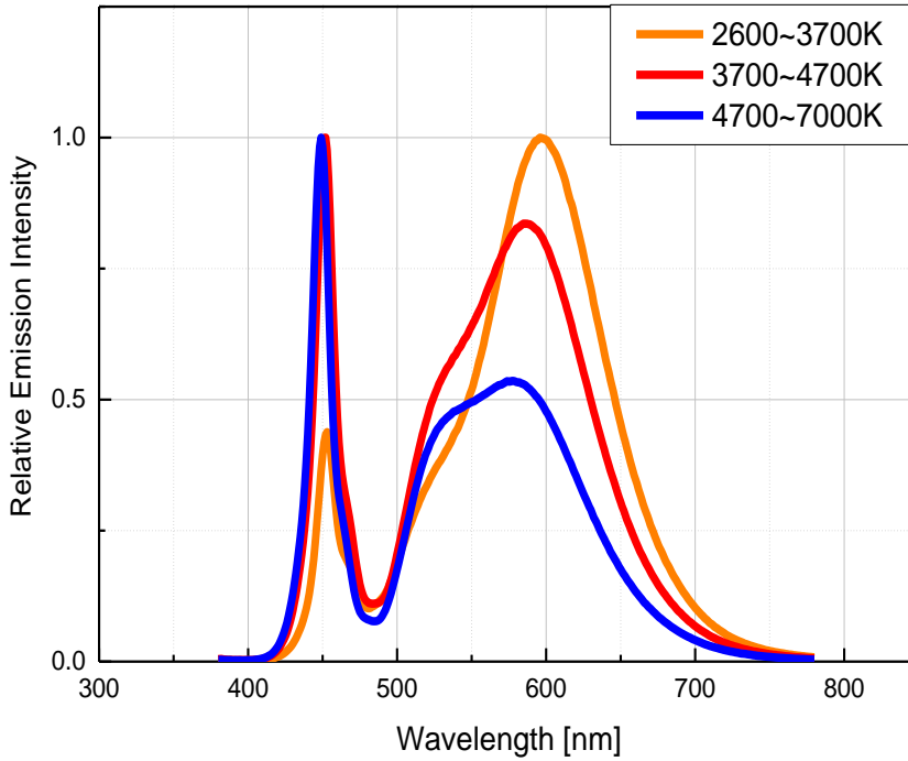
Fig 1. Color Spectrum, T_j=25^\circ\text{C} , I_F=65\text{mA}
