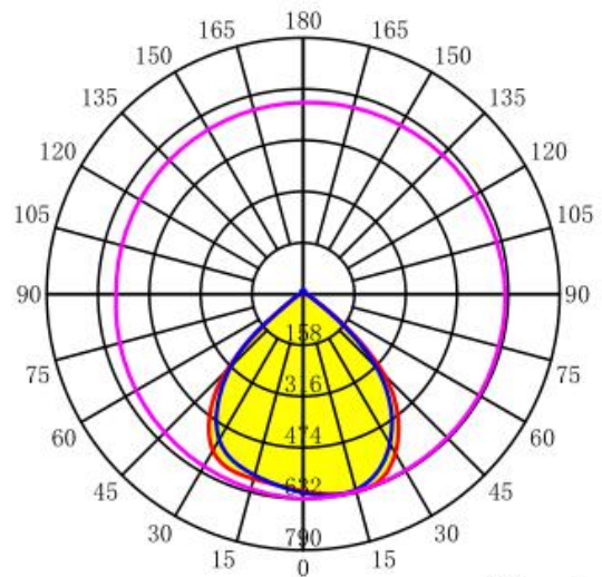
配光曲线
