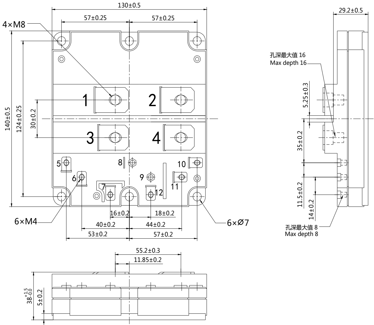
图11. 模块外观尺寸
