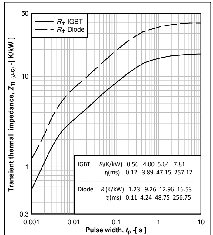
图10. 瞬态热阻抗曲线
