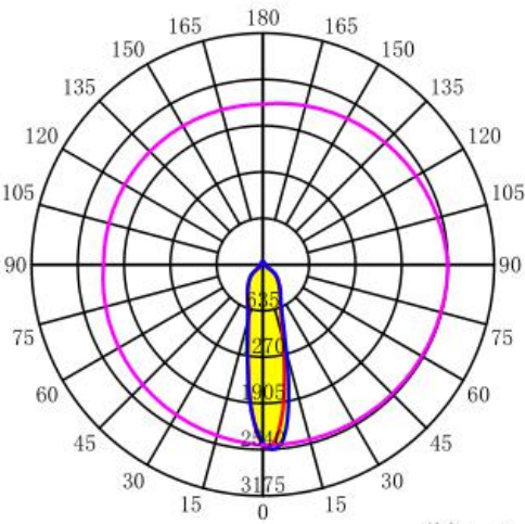
配光曲线
