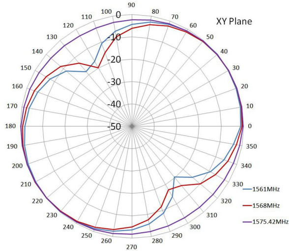
GPS Antenna
