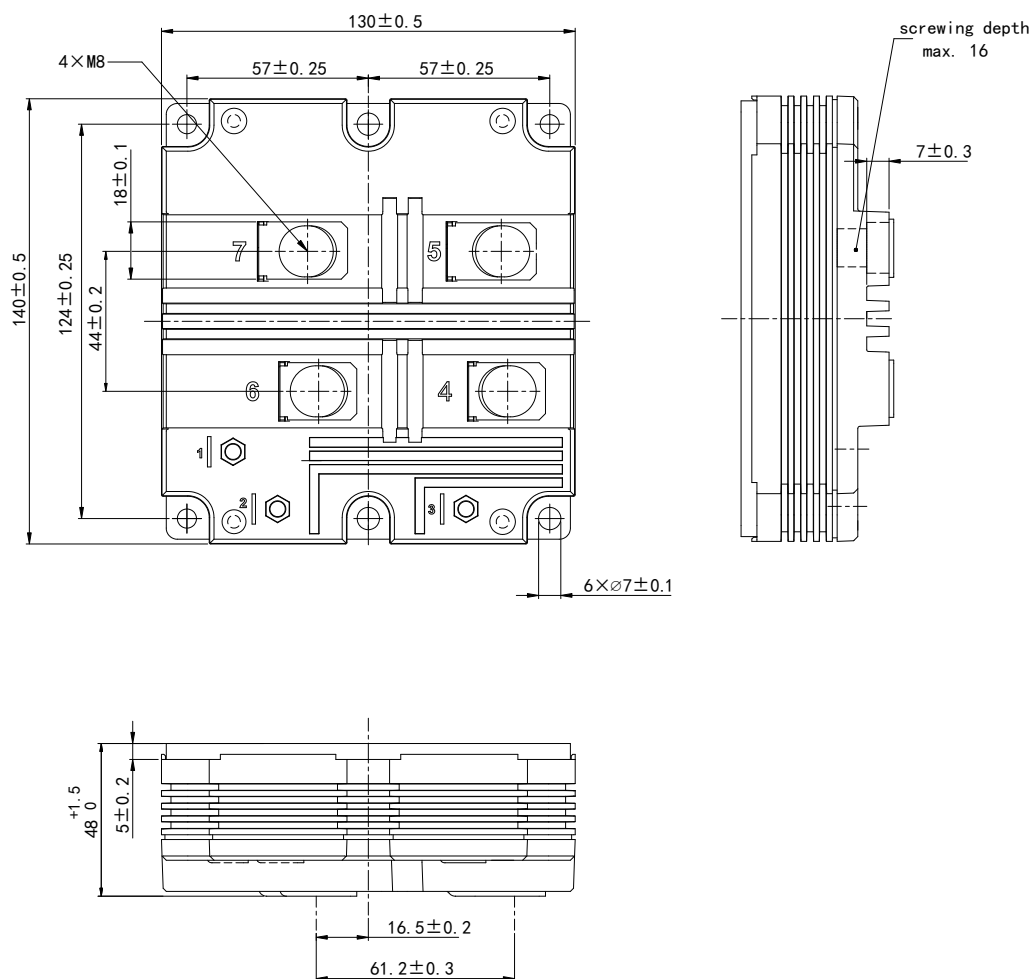
图 10. 模块外观尺寸
