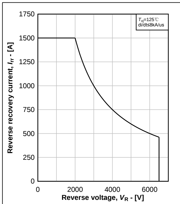
图 8. 二极管反偏安全工作区
