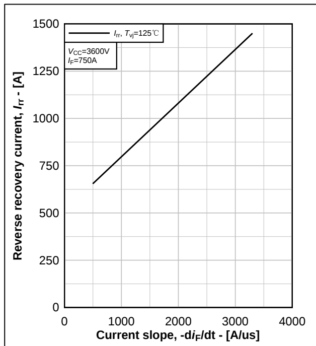
图 7. 反向恢复电流典型曲线, I_{rr} = f(-di_F/dt)
