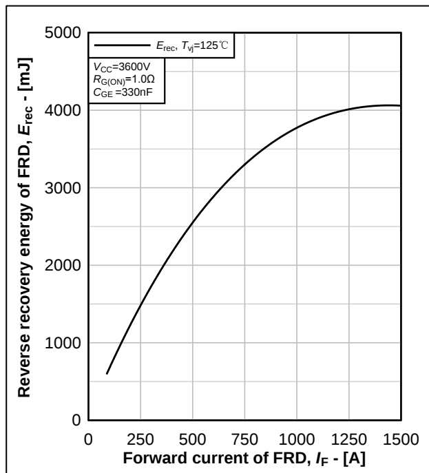
图 4.反向恢复能耗典型曲线, E_{rec} = f(I_F)
