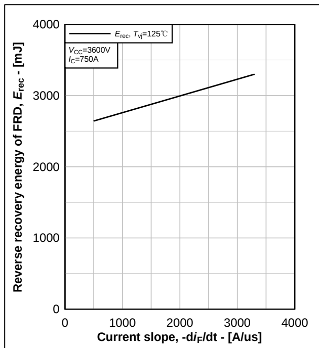
图 5.反向恢复能耗典型曲线, E_{rec} = f(-di_F/dt)
