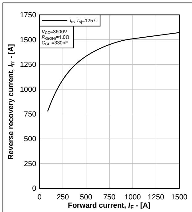
图 6.反向恢复电流典型曲线, I_{rr} = f(I_F)
