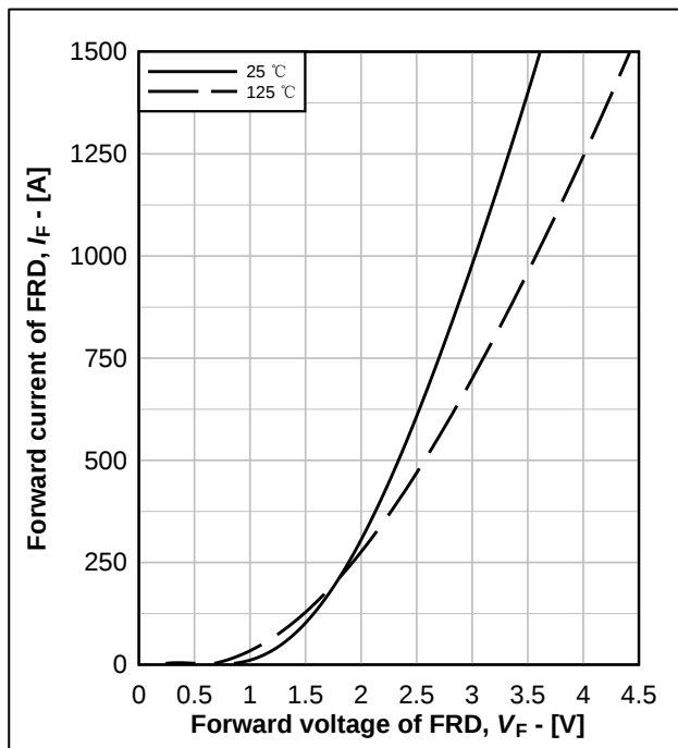
图 3.输出特性典型曲线, I_F = f(V_F)
