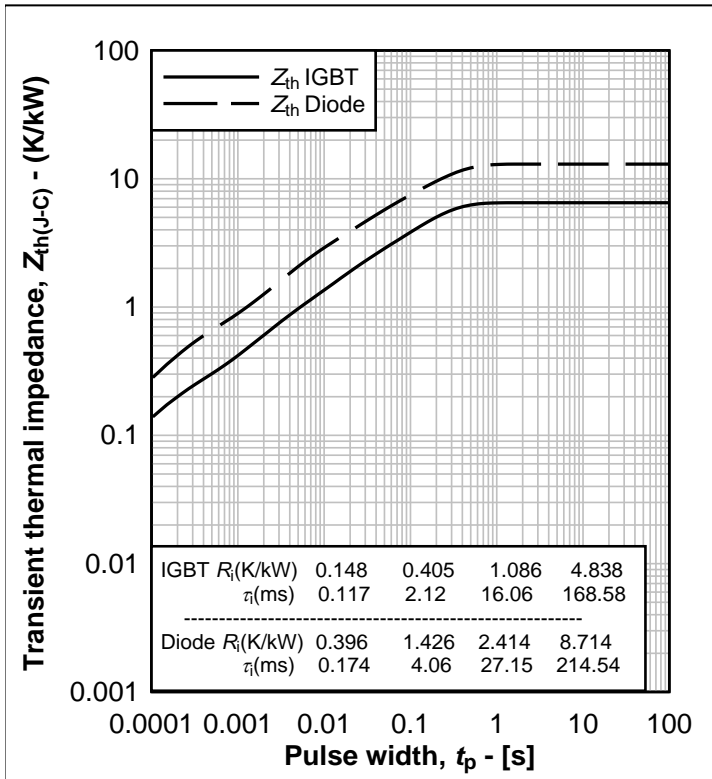
图9. 瞬态热阻抗曲线
