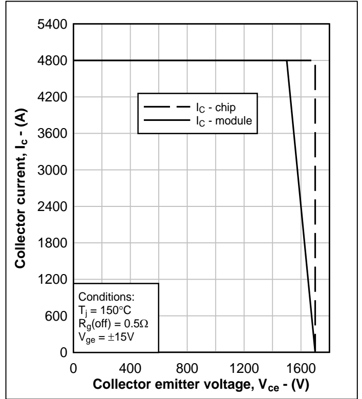
图8. 反偏安全工作区
