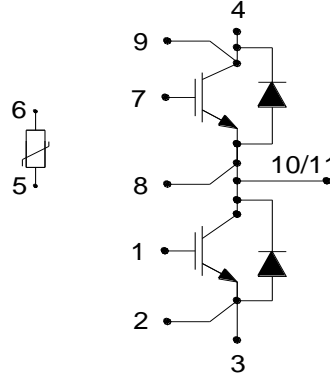
1. 电路结构
