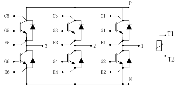
图 1. 电路结构
