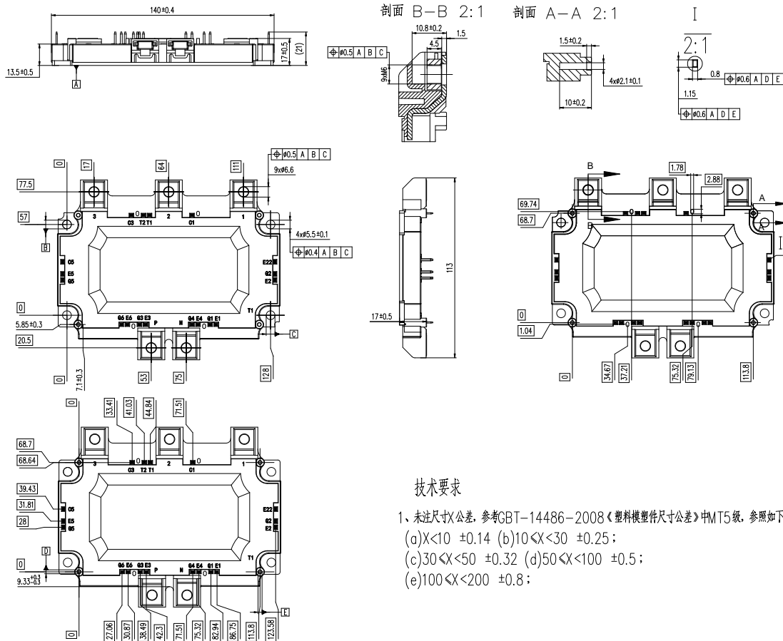
图 15. 模块外观尺寸
