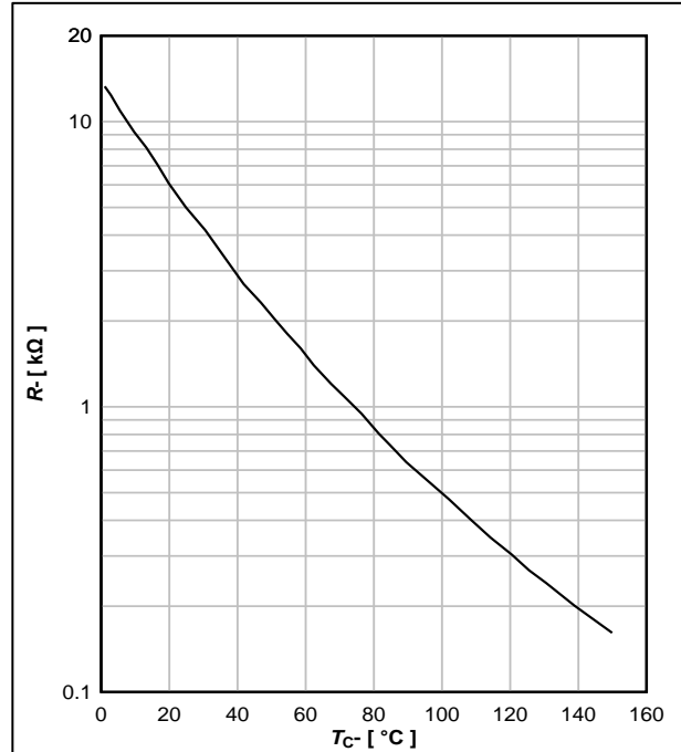
图 12. 热敏电阻典型特性曲线, R = f(T_C)
