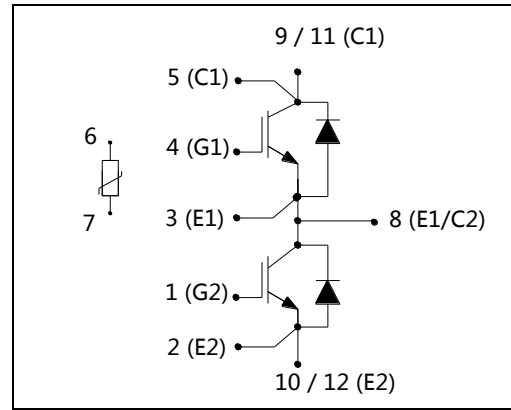
图 1. 电路结构
